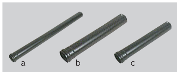
a.直管(1m) サイズ: \phi 80 \times 1000\text{m/m} b.直管(50cm) サイズ: \phi 80 \times 500\text{m/m} c.直管(25cm) サイズ: \phi 80 \times 250\text{m/m}
