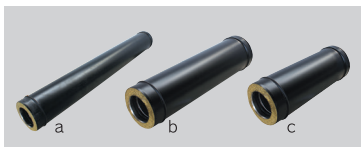
a.直管(96cm) サイズ: \phi 130 \times 960\text{m/m} b.直管(46cm) サイズ: \phi 130 \times 460\text{m/m} c.直管(32cm) サイズ: \phi 130 \times 320\text{m/m}
