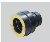
異径ソケットY型 サイズ: \phi 80 \times \phi 130\text{m/m}
